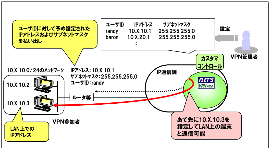
図1-7 LAN型払い出し
